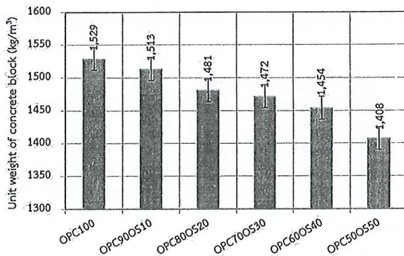
รูปที่ 2 Unit weight of concrete block
