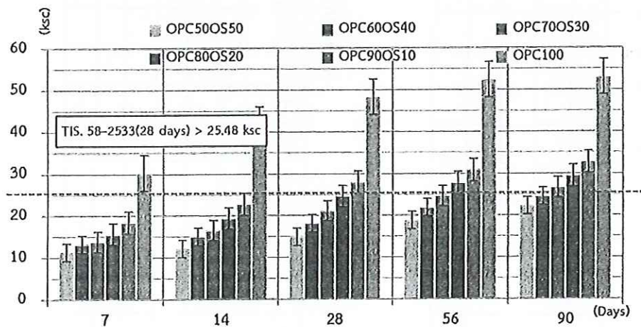
รูปที่ 3 Compressive strength of concrete block
